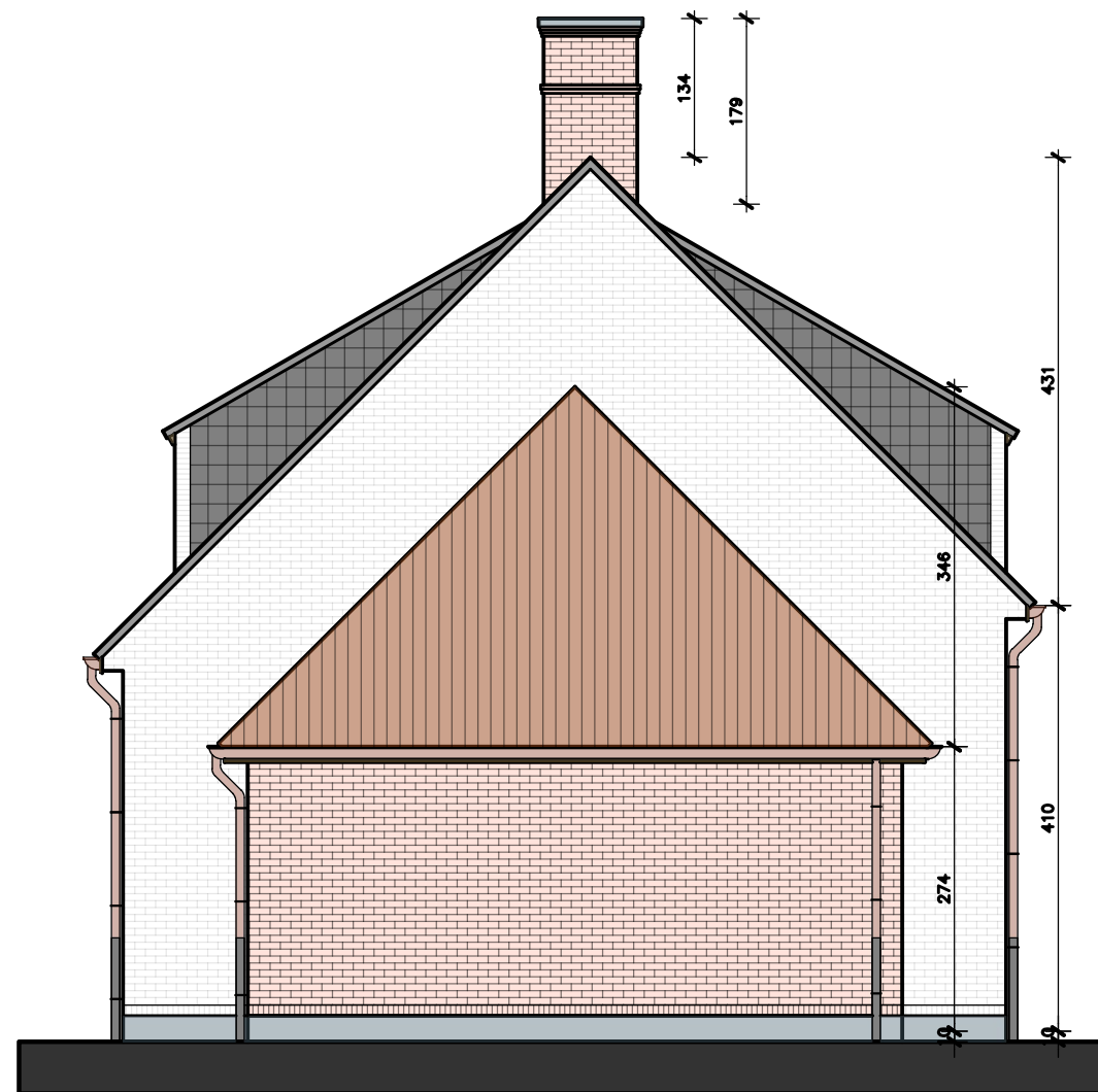
Zijgevel Links Woning 06
