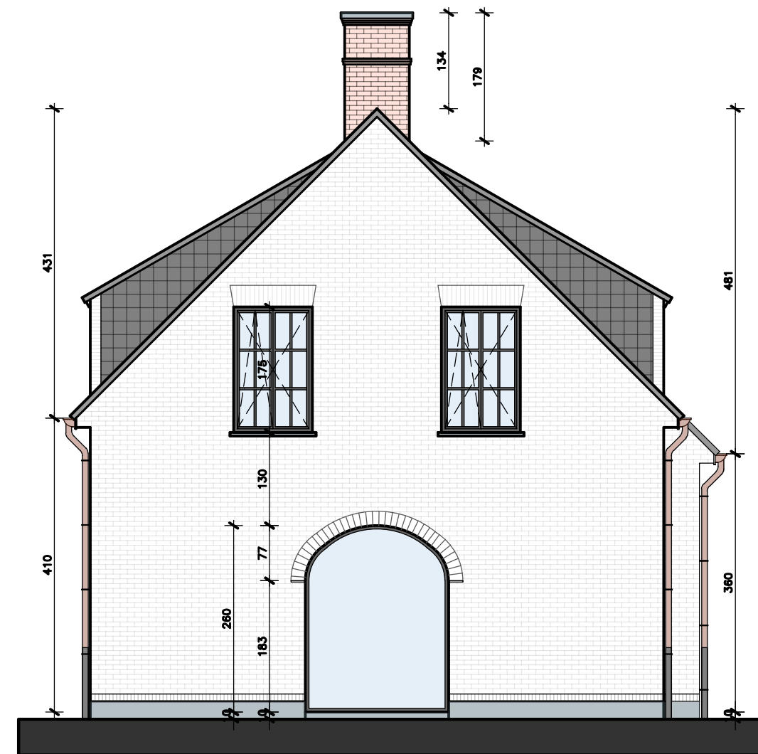
Zijgevel Rechts Woning 06
